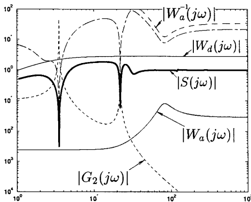
Figure 2: Design result of controller ( |S(j\omega)| , |G_2(j\omega)| , |W_d(j\omega)| , |W_a(j\omega)| )
