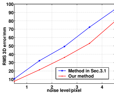
Fig. 2. 3D Error
