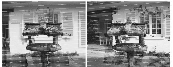
FIG. 2 – Le sous-échantillonnage de la mise en correspondance quasi-dense (décrit en section 4) est représentés par un ensemble de croix noires dans les deux images. Ces appariements bien répartis sont utilisé pour estimer la matrice fondamentale, dont certaine des lignes épipolaires sont dessinées.
