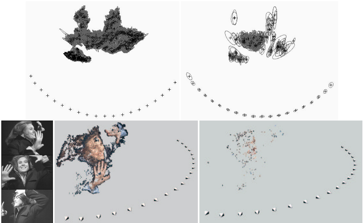
FIG. 4 – Reconstructions QUASI (gauche) et EPARS (droite) pour Lady. Les ellipsoïdes à 90% pour l'ajustement de faisceaux final sont zoomés 4 fois pour aider la visualisation. Trois images de la séquence Lady sont aussi données.
