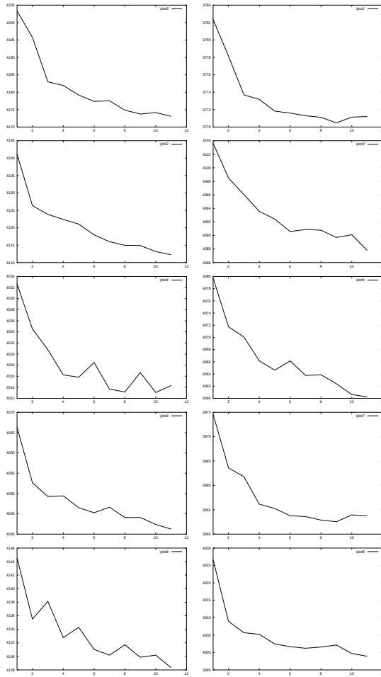
FIG. 13 – Convergence des dix modèles : Le coût moyen des données d'apprentissage ( -\log(P) ) est tracé en fonction du nombre d'itérations dans le calcul du modèle.
