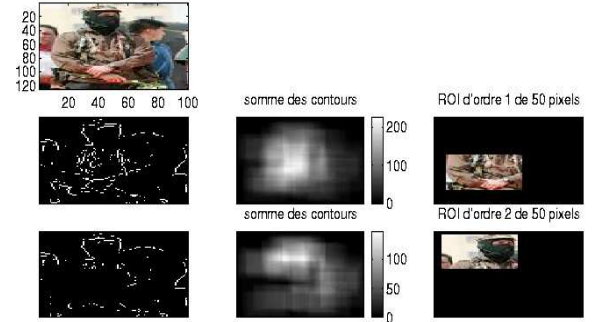
FIG. 3 – Sélection des 2 premières régions locales d'intérêts (ROI) d'une image par détection des contours par la méthode de Canny et par maximisation des sommes des contours par région. Photo ©Editing.
