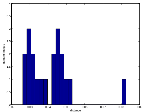
FIG. 6 – Distribution des distances \delta_{V_A} pour chaque image trouvée par la requête sur Google. Cette distribution est bimodale, ce qui permet de considérer que les images du premier groupe (à gauche de 0.04) sont adéquates à la requête, à droite non.
