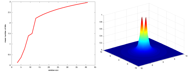
FIG. 3: À gauche : évolution de la mesure d' ELM (en bits) en fonction de la taille de la fenêtre expérimentale choisie pour l'estimation des probabilités marginales sur l'image de Lena. À droite : facteur de pondération multiéchelle finalement choisi sur une fenêtre de rayon 21 \times 21 pixels.
