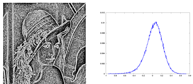
FIG. 4: À gauche : image des singularités ; un pixel est d'autant plus clair que son exposant de singularité locale est petit. À droite : histogramme de distribution des exposants de singularité.
