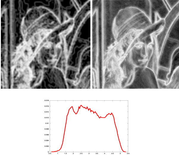
FIG. 2: En haut : EL et ELM calculées sur l'image de Lena ; à gauche, l'entropie est estimée sans pondération sur des fenêtres de taille 10 \times 10 ; à droite, on introduit une pondération multiéchelle sur des fenêtres de taille 21 \times 21 (cf. section 2.3). En bas : distribution de l' ELM sur l'image.
