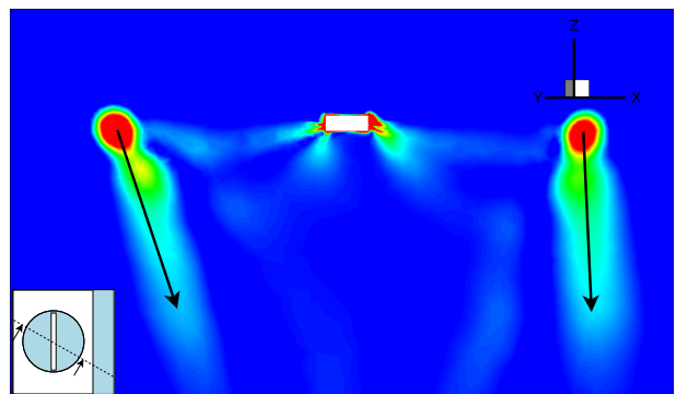
(d) Near-wall (2c gap) 30°/210° plane
